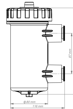
Előremenő/visszatérő szelep
