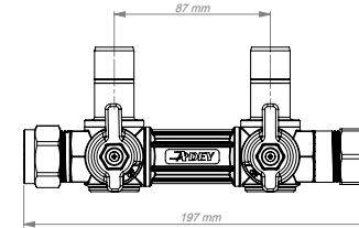
Előremenő/visszatérő szelep
