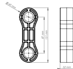
Távtartó gyűrű
