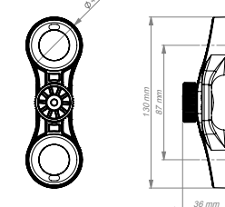
Szorító gyűrű
